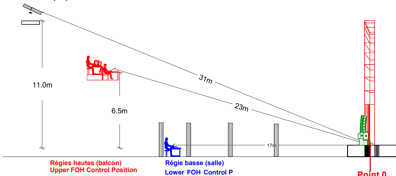
Vue de coupe - Section View
